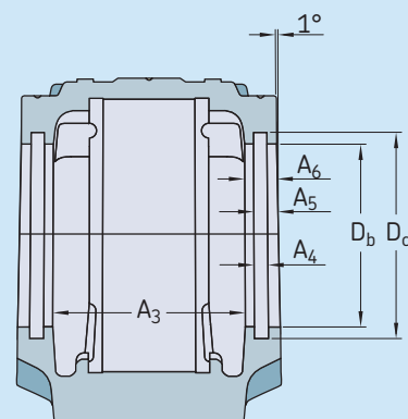
Seal groove dimensions
