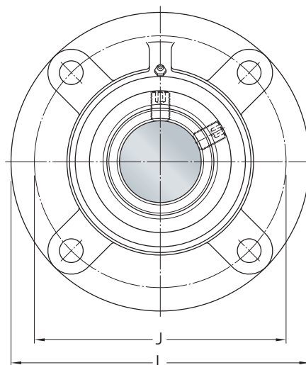
FYRP
